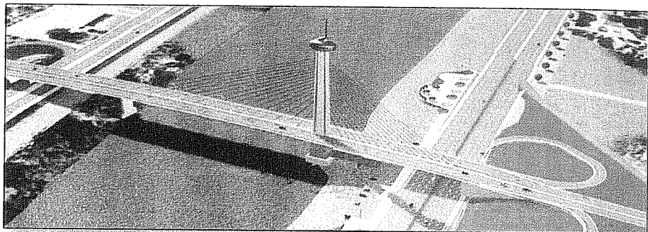
Dados técnicos: Ponte estaiada, com 379 m de extensão e 28,90 m de largura, duas pistas, cada uma com 3 faixas de tráfego; vão livre sobre o rio de 160 metros.
